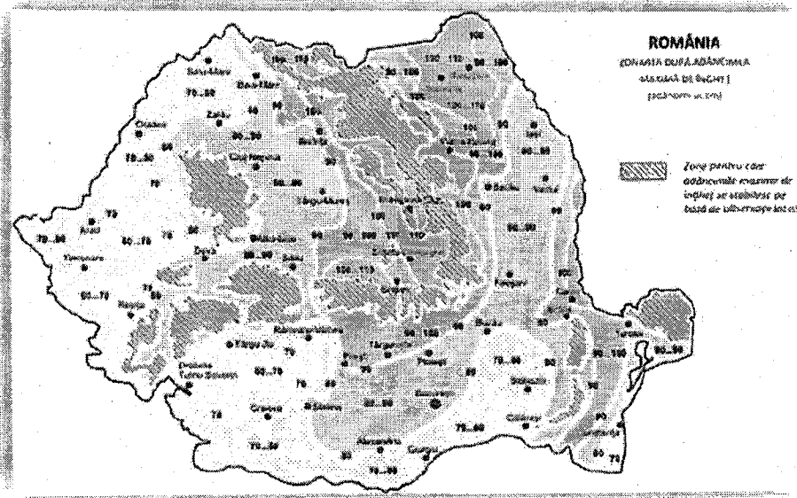
Figura 1 - Zonarea teritoriului Romaniei dupa adancimea de inghet
