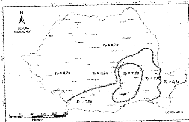
Figura 4 - Zonarea teritoriului în termeni de perioadă de control (colt), T_c , a spectrului de răspuns
